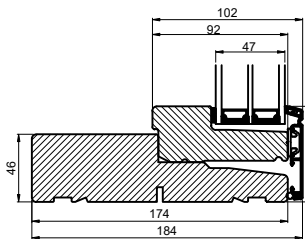
Sidekarme/ sideframe
