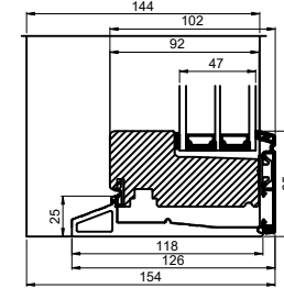
Med glasfibertrin/ With fiberglass threshold
