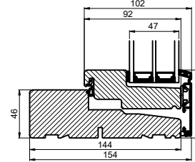
Med hårdttrætrin/ With hardwood threshold
