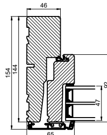
Vindue og vinduesdør/ Window and window door
