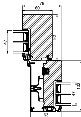
Vandret snit A/ Horizontal section A
