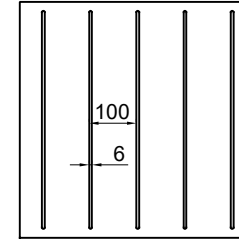
Fyldning med alu spor type 40 (variabel C-C)
