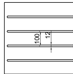
Fyldning med vandret alu spor (100 mm C-C)
