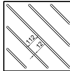
Fyldning med skrå alu spor (112 mm C-C)
