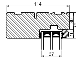
Lodret snit A
